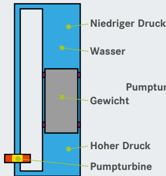
Außen liegende Pumpturbine
